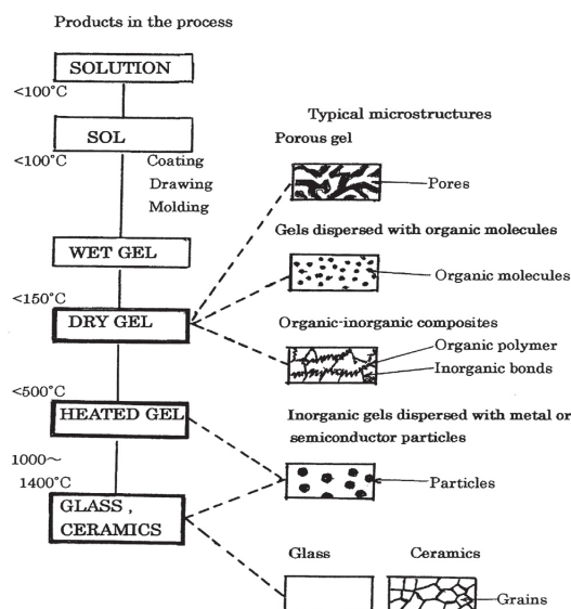
شکل ۱- مراحل فرایند سل-ژل و ریز ساختار محصول نهایی را نشان می‌دهد [۳].
