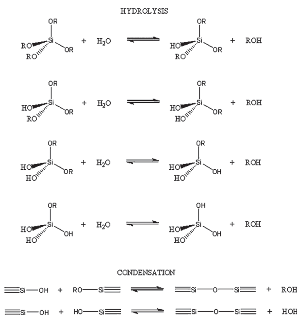
شکل ۲- مراحل هیدرولیز و تراکم را که در ساخت سیلیکا سل-ژل نقش دارند را نشان می‌دهد.
