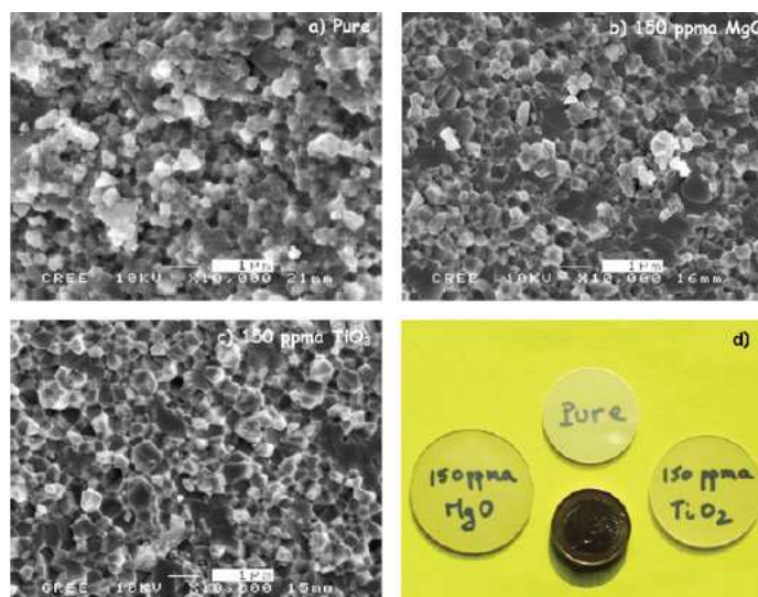
شکل ۳- ریزساختار پس از زینتر به مدت ۳ ساعت در دمای 1250^{\circ}\text{C} و HIP به مدت ۱۵ ساعت در 1250^{\circ}\text{C} (a) خالص (b) ۱۵۰ ppm MgO (c) ۱۵۰ ppm \text{TiO}_2 و (d) تصویر پنجره‌های پولیش شده [۲۲]
