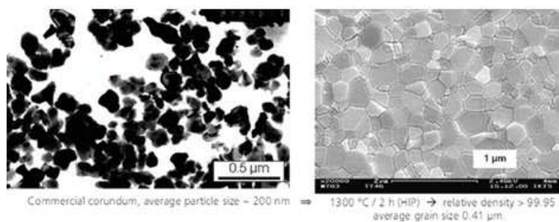
شکل ۵- تصویر SEM پودر آلومینای اولیه و ریزساختار حاصل پس از HIP به مدت ۲ ساعت در 1300^{\circ}\text{C} [۳۴]
