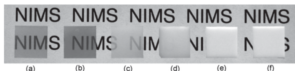
شکل ۷- آلومینای زینتر شده به روش SPS با افزودن 0.125\% وزنی MgO و نرخ گرمایش (a) 2^{\circ}\text{C}/\text{min} (b) 5^{\circ}\text{C}/\text{min} (c) 10^{\circ}\text{C}/\text{min} (d) 25^{\circ}\text{C}/\text{min} (e) 50^{\circ}\text{C}/\text{min} (f) 100^{\circ}\text{C}/\text{min} [۳۸].
