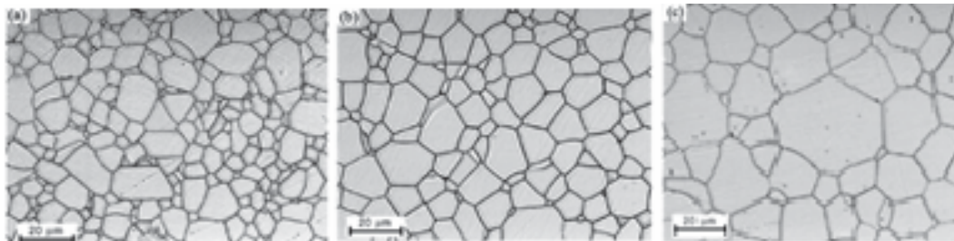
شکل ۸- ریزساختار آلومینا با ۰/۵ درصد وزنی MgO. زینتر با استفاده از ماکروویو در دمای ۱۷۵۰°C، نرخ حرارت دهی ۱۰۰°C/min برای مدت زمان (a) ۱۵، (b) ۳۰ و (c) ۴۵ دقیقه، صورت گرفته است [۴۲].
