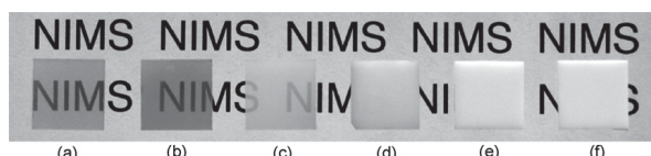
شکل ۷- آلومینای زینتر شده به روش SPS با افزودن 0.125\% وزنی MgO و نرخ گرمایش (a) 2^{\circ}\text{C/min} (b) 5^{\circ}\text{C/min} (c) 1^{\circ}\text{C/min} ، (d) 25^{\circ}\text{C/min} (e) 50^{\circ}\text{C/min} (f) 100^{\circ}\text{C/min} [۳۸].
