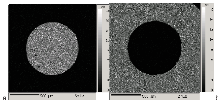
شکل ۷- تصویر پرتو X از فیبر تنگستن و زمینه شیشه فلز با استفاده از (a) W La (b) Zr La [۹]
