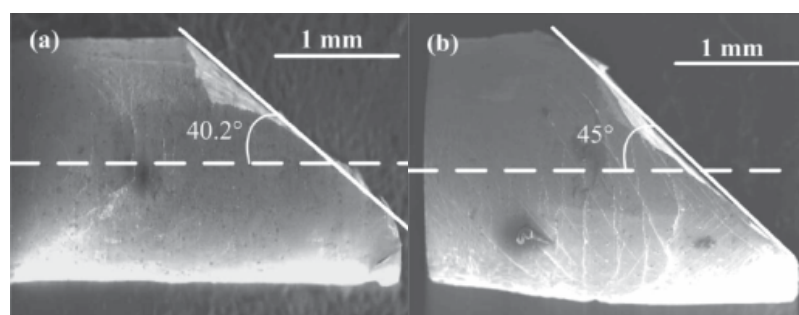
شکل ۲- تصویر SEM از مقطع شکست نمونه آلیاژ آمورف (a) \text{Cu}_{50}\text{Zr}_{50} ، (b) \text{Cu}_{47.5}\text{Zr}_{47.5}\text{Al}_5 پس از آزمایش فشار سرد [۶]
