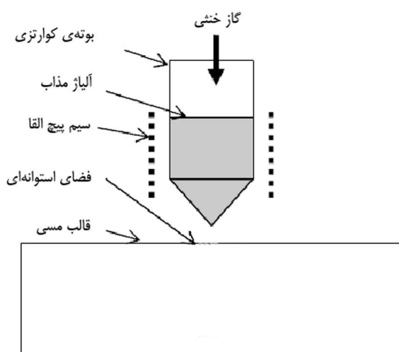
شکل ۴- نمایش سیستم استفاده شده در ساخت شیشه فلز حجمی [۹]
