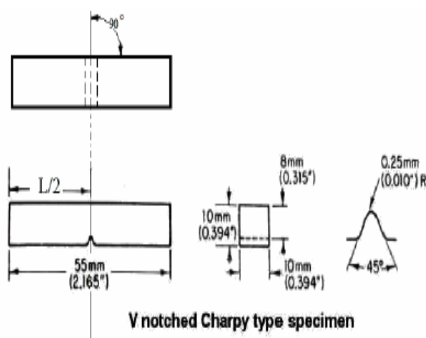
شکل ۱- ابعاد نمونه‌ی آزمایش ضربه شاریپی بر اساس استاندارد ASTM A۳۷۰
