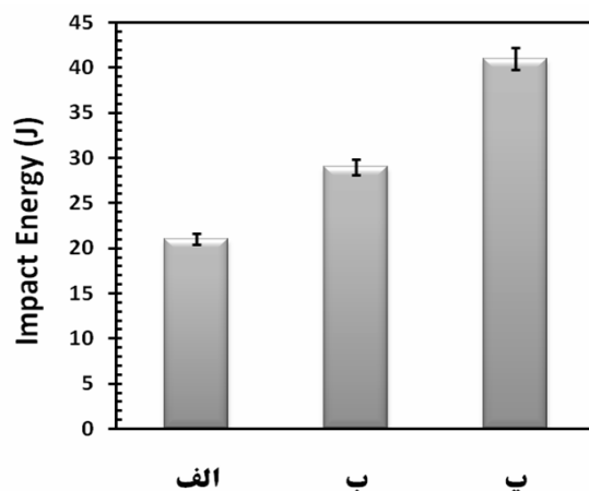
شکل ۶- متوسط نتایج آزمایش ضربه شاری با حداقل ۳ بار تکرارپذیری در نمونه‌های ریخته‌گری شده در قالب: (الف) ماسه سیلیسی، (ب) ماسه الیوینی، (پ) ماسه کرومیتی.
