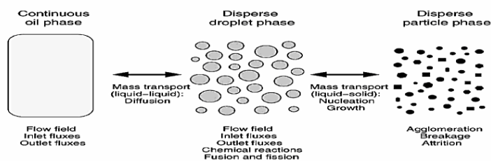
شکل (۲) سازوکار پیشنهادی جهت تشکیل نانو ذرات از محلول میکرومولسیون [۹].
