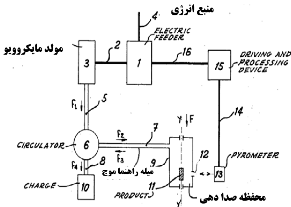
قرارگیری دستگاه‌ها در اختراعتفجوشی سرامیک‌ها با مایکروویو
