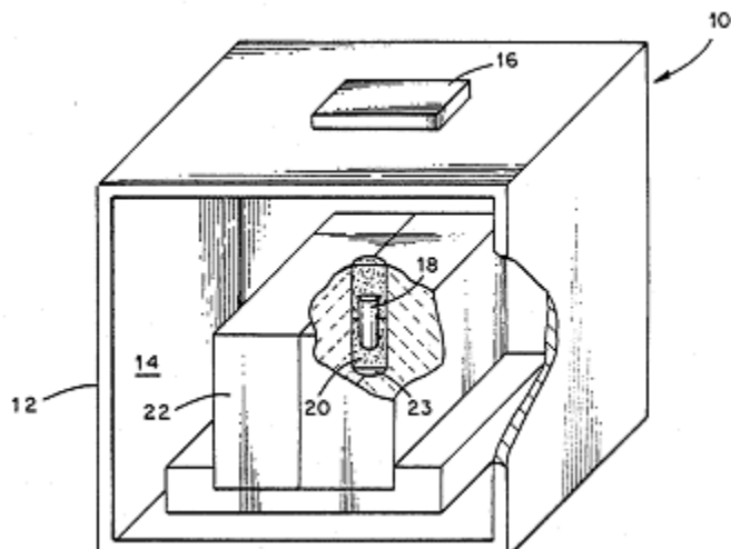
ست آپ دستگاه برای اختراع در مورد روش تفجوشی و عملیات حرارتی (نمونه با شماره ۱۸ و ماده در برگزیده با شماره ۱۱/۳۰).
