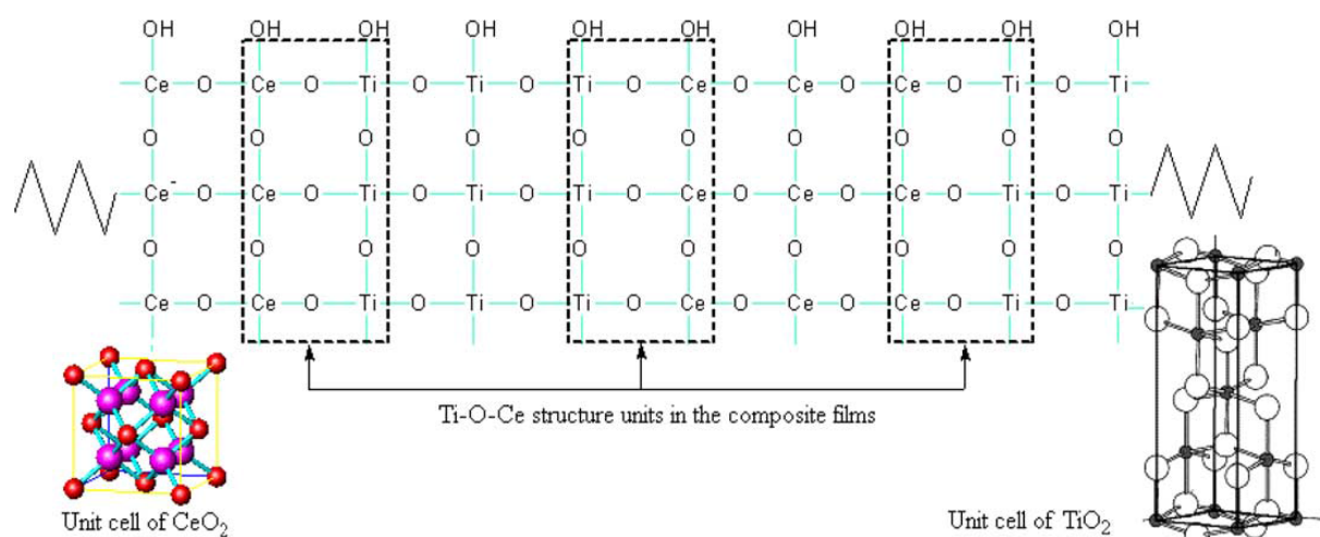
شکل ۴- نموداری از ساختار فیلم‌های کامپوزیتی و سلول‌های واحد TiO 2 و CeO 2 .
