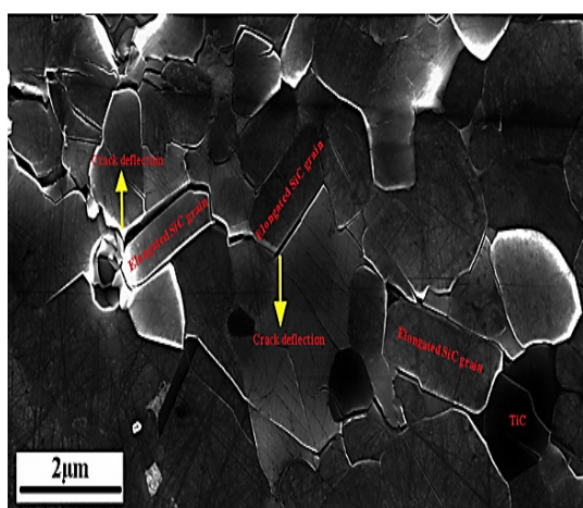
شکل ۳- مسیر ترک در امتداد دانه‌های کشیده شده‌ی SiC [۱۶].
