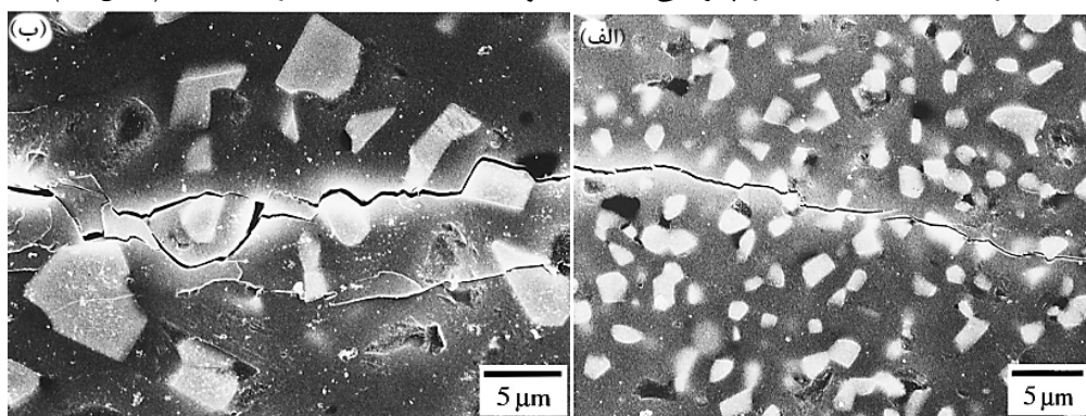
شکل ۱۲- تصاویر SEM از مسیر اشاعه ترک در کامپوزیت‌های زمینه SiC حاوی ۲۰ درصد حجمی TiB 2 . (الف) نمونه‌های زینتر شده در دمای ۲۱۰۰°C به وسیله بدون فشار و HIP، (ب) نمونه‌های زینتر شده در دمای ۲۲۰۰°C به وسیله بدون فشار و HIP [۲۱].
