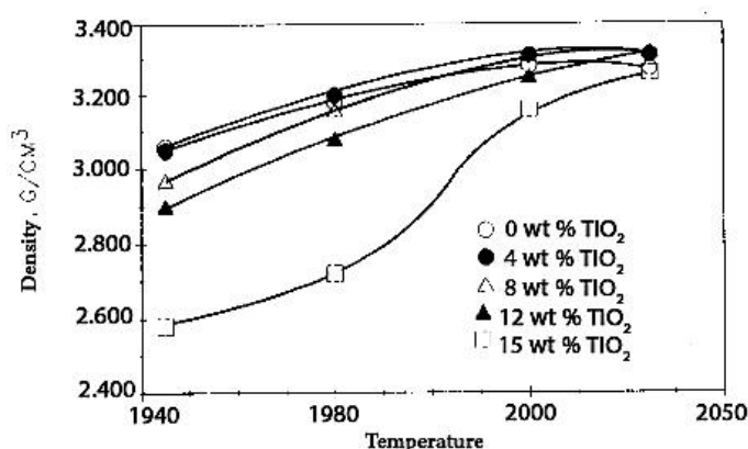
شکل ۱- تغییرات چگالی با دمای زینتر برای مقادیر مختلف TiO_2 [۱۵]
