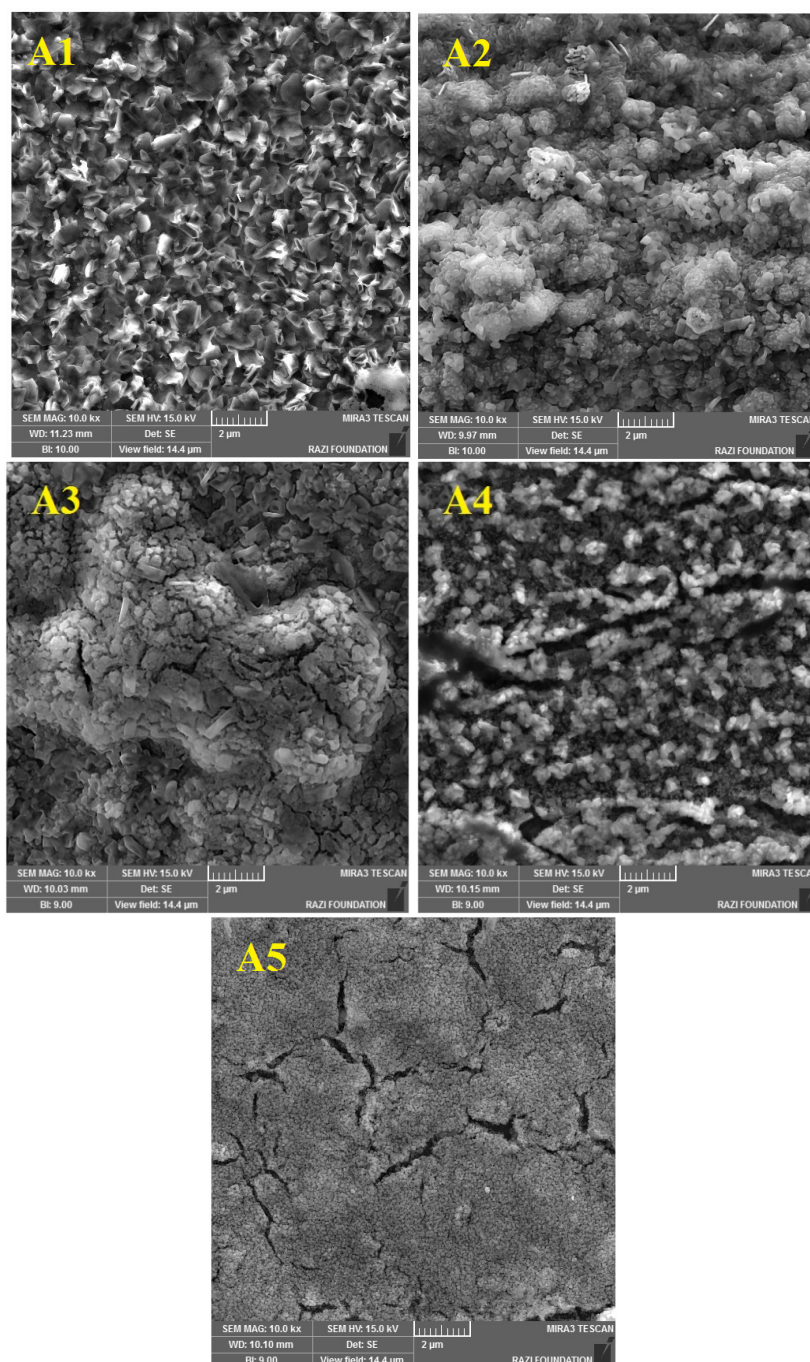
شکل ۳- تصاویر SEM از سطح نانو فیلم‌ها پس از عملیات حرارتی در دمای 700^\circ\text{C} .
