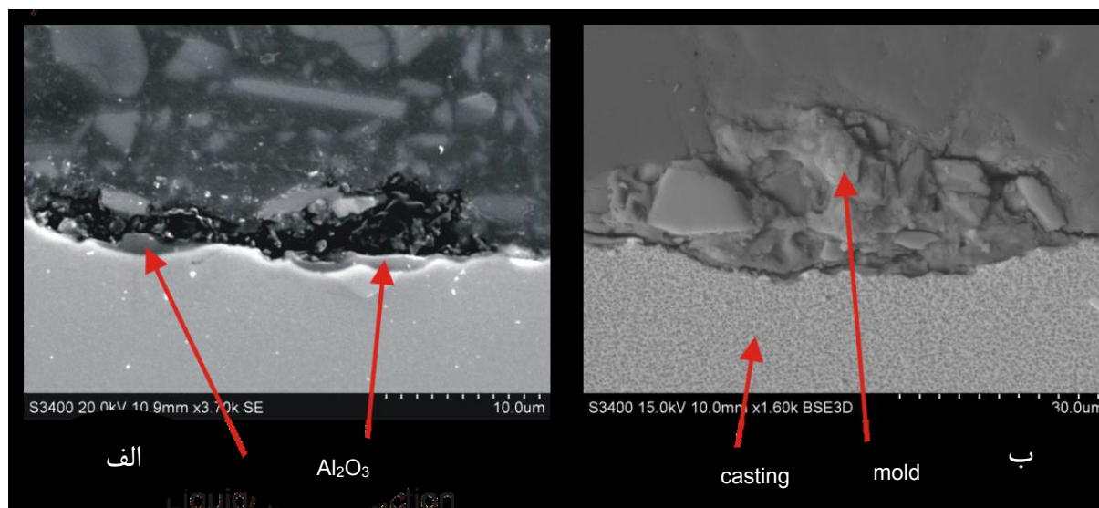
شکل ۱- واکنش بین قالب و مذاب ریخته گری شده. (الف) تشکیل یک لایه آلومینا در اثر واکنش بین سیلیکا از قالب سرامیکی و آلومینیوم موجود در مذاب. (ب) تشکیل لایه اکسیدی در سطح تماس قطعه و قالب [۹].
