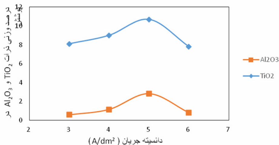
شکل ۴- تاثیر دانشیه جریان بر درصد وزنی ذرات TiO_2 و Al_2O_3 پوشش
