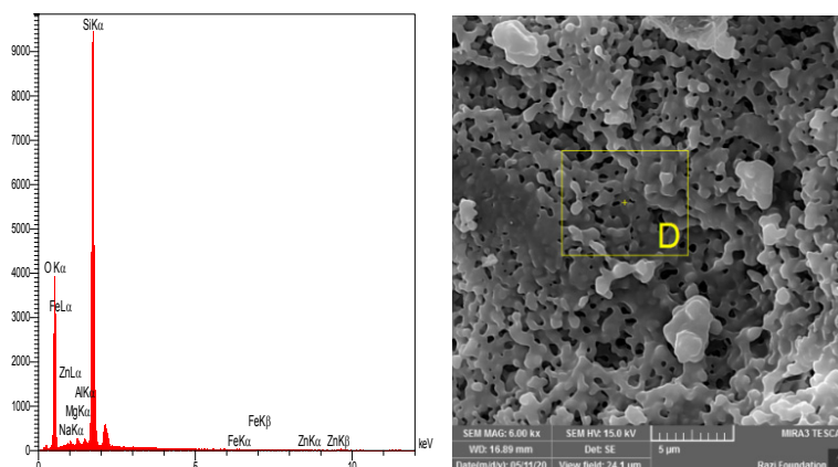
شکل ۵- تصویر میکروسکوپ نیروی الکترونی از سطح لعب یک استوپر تجاری بعد از پیشگرم کردن به همراه آنالیز EDS از نقطه D. قسمت اعظم لعب را \text{SiO}_2 تشکیل می‌دهد.
