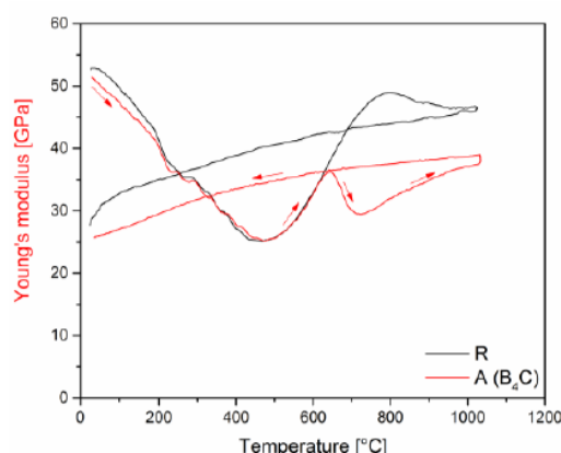
شکل ۳- منحنی مدول یانگ دیرگداز \text{Al}_2\text{O}_3\text{-C} حاوی آنتی اکسیدان کاربید بور [۵]
