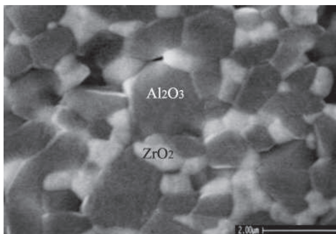
شکل ۳- تصویر میکروسکوپ الکترونی روبشی (SEM) ریزساختار کامپوزیت آلومینا با ۲۰ درصد حجمی زیر کونیا که در دمای 1650^{\circ}\text{C} درجه سانتی گراد سینتر شده است ( نمونه در دمای 1500^{\circ}\text{C} و به مدت ۲۰ دقیقه اچ حرارتی شده).
