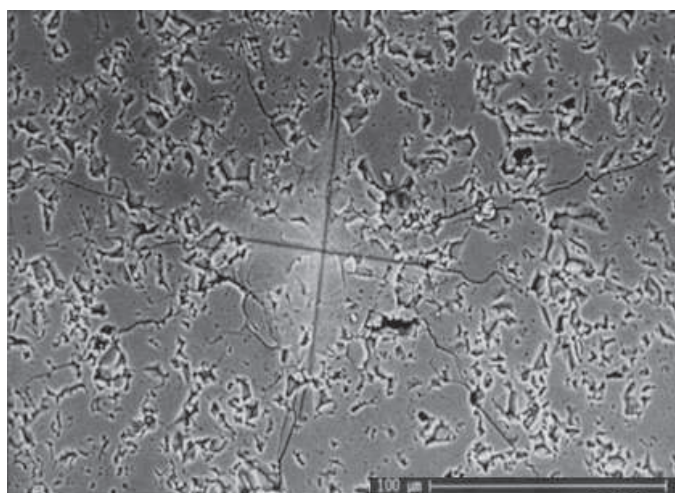
شکل ۸- تصویر میکروسکوپ الکترونی روبشی (SEM) از ترک‌های پدید آمده توسط فرو رونده ویکرز با نیروی ۱۰۰ نیوتن بر روی نمونه آلومینایی که در دمای ۱۶۵۰ درجه سانتی‌گراد سینتر شده است. (نمونه در دمای 1300^{\circ}\text{C} و به مدت ۳۰ دقیقه اچ حرارتی شده).
