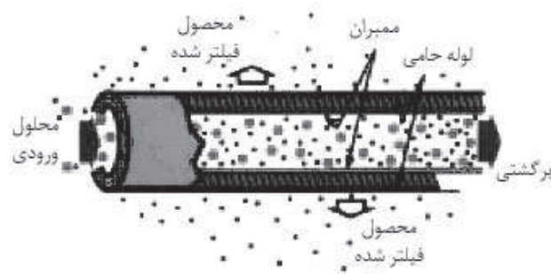
شکل ۵- نمای شماتیک ممبران لوله ای شکل [۶]
