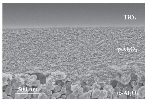
شکل ۴- مقطع عرضی ممبران شامل لایه آمورف \text{TiO}_2 در سطح، لایه میانی \gamma\text{-Al}_2\text{O}_3 و پایه [\alpha\text{-Al}_2\text{O}_3]
