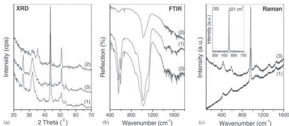
شکل ۲- (الف) الگوهای XRD، طیف‌های (ب) FTIR و (ج) رامان لایه HA رشد یافته بر پیش ماده مایع در 26^{\circ}\text{C} و 37^{\circ}\text{C} پس از تابش اولیه لیزر.
