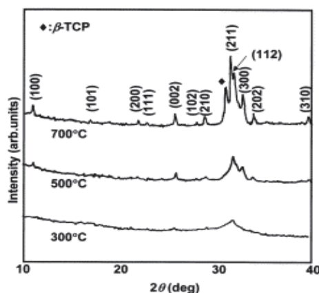
شکل ۵- الگوی پراش پرتو X پوشش HA بر زیر لایه (۱۰۰) Si که در دماهای مختلف پخت شده است.
