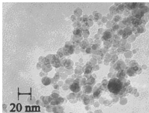
شکل ۹- میکروگراف TEM نانوپودر \text{TiO}_2 سنتز شده به روش CF-CVC [۱۸]
