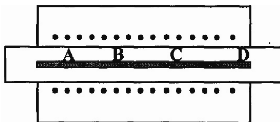
شکل ۸- شماتیکی از محل‌های جمع‌آوری ذرات داخل راکتور CVC [۱۷]
