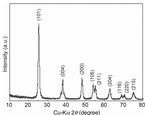
شکل ۴- الگوی XRD نمونه‌ی \text{TiO}_2 که به مدت ۴ ساعت شده در دمای 400^\circ\text{C} تکلیس شده است [۷]
