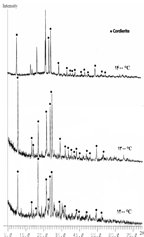
شکل ۱۰- تحولات فازی کوردیریت با استفاده از تالک فرانسه و با کربنات باریم ۴٪ در درجه حرارت‌های مختلف
