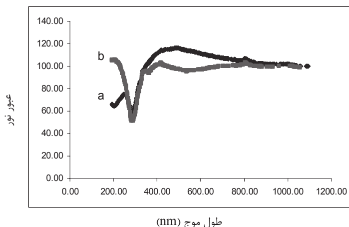
شکل ۲- نمودارهای درصد عبور نور بر اساس طول موج نمونه عملیات حرارتی شده در دمای ۴۵°C و ۶۸°C (a) از قبل روشن (b) بعد از ۳ دقیقه تابش پرتوهای UV
