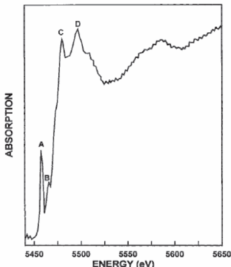
شکل ۱- آزمون XANES برای یک نمونه رنگدانه آبی پایه زیرکسی [۹]
