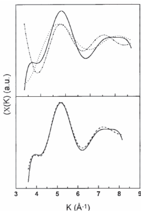
شکل ۳- نمایشی از نتیجه آزمون EXAFS در حالت‌های مختلف [۸] آب پایه زیرکونی بر اساس عدد موج [K(\text{\AA}^{-1})] [۹]
