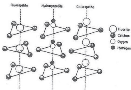
شکل ۱- مقایسه موقعیت اتم‌های \text{OH} ، \text{F} و \text{Cl} در مرکز مثلث \text{Ca} در ساختار HA [۱]
