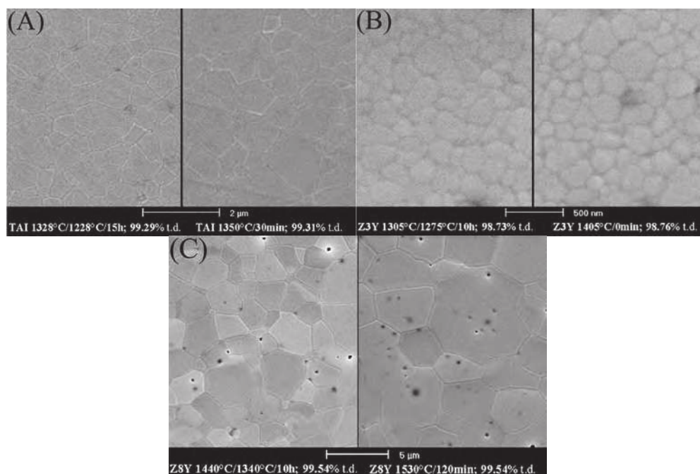
شکل ۸- تصاویر میکروسکوپ الکترونی روبشی نمونه‌های سینتر شده به‌روش معمولی و دو مرحله‌ای (a) آلومينا (b) ايتريا ۳٪ مولى زیرکونیا (c) ايتريا ۸٪ مولى زیرکونیا [۱۳]
