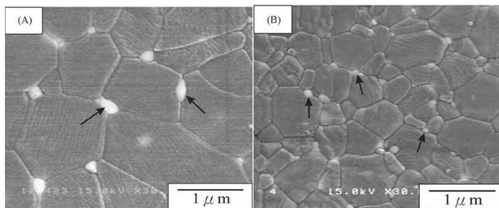
شکل ۱۰- ریزساختار آلومینای کاملاً متراکم تهیه شده از (A) سینتر با سرعت حرارت دهی ثابت ( 1600^{\circ}\text{C}/4\text{h} ) و (B) سینتر دو مرحله‌ای ( T_1=1450^{\circ}\text{C} , T_2=1350^{\circ}\text{C}/12\text{h} ). داده‌های روشن که با فلش مشخص شده فاز زیرکونیا می‌باشد [۳].
