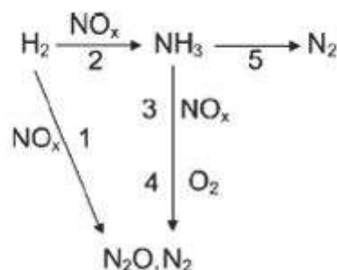
شکل ۳- مجموعه واکنش‌ها حین احیاء \text{NO}_x ذخیره شده با \text{H}_2 که شامل پنج مرحله است [۱۳].
