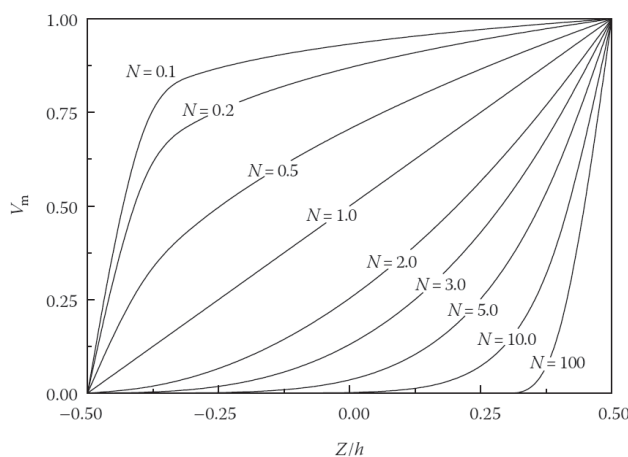
شکل ۱۰- توزیع فلز در ضخامت برای مقادیر مختلف توان کسر حجمی (N) [۲۳]
