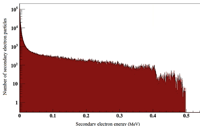
شکل ۱۷: نمایش طیف انرژی الکترون ثانویه خروجی از حفاظ P6 به ازای 10^6 ذره فرودی با انرژی ۰/۵ مگاالکترون‌ولت
