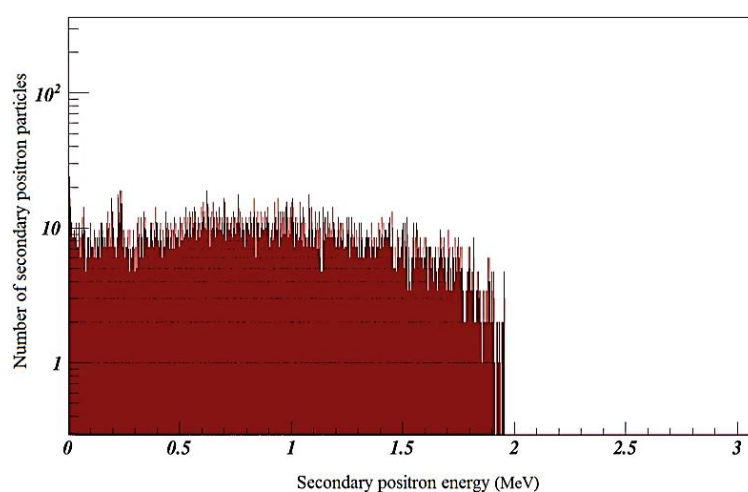
شکل ۱۸: نمایش طیف انرژی پوزیترون ثانویه خروجی از حفاظ P6 به ازای 10^6 ذره فرودی با انرژی ۳ مگاالکترون‌ولت
