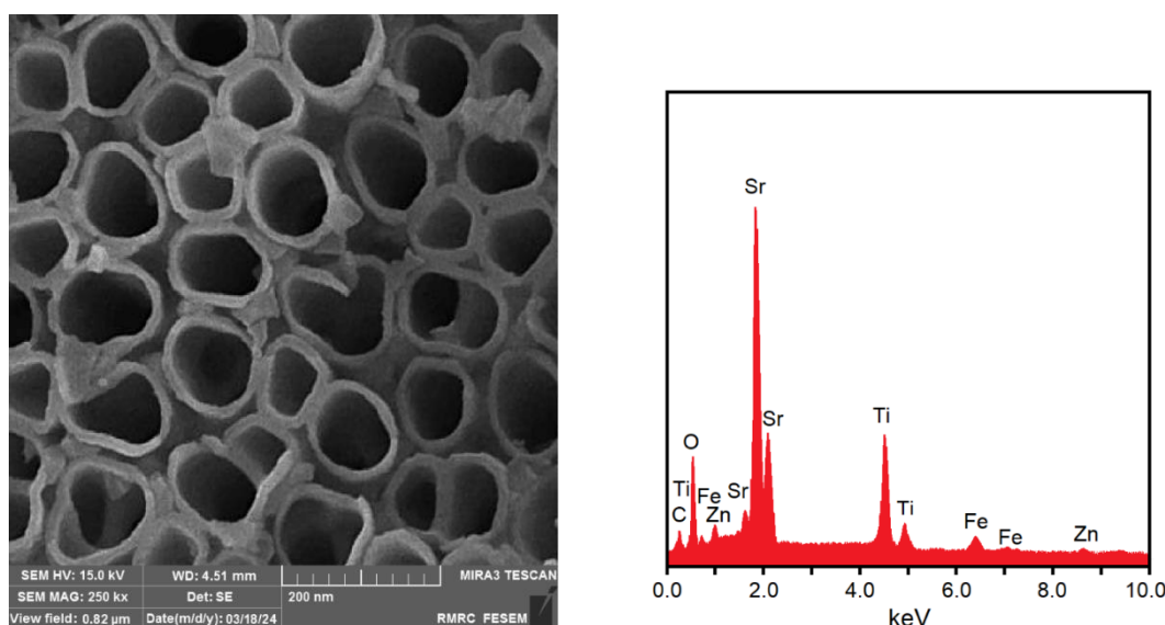
شکل ۲: الف) تصویر FESEM مربوط به نانولوله‌های تیتانات استرانسیم دوپ‌شده با روی و آهن ب) آنالیز EDS نمونه
