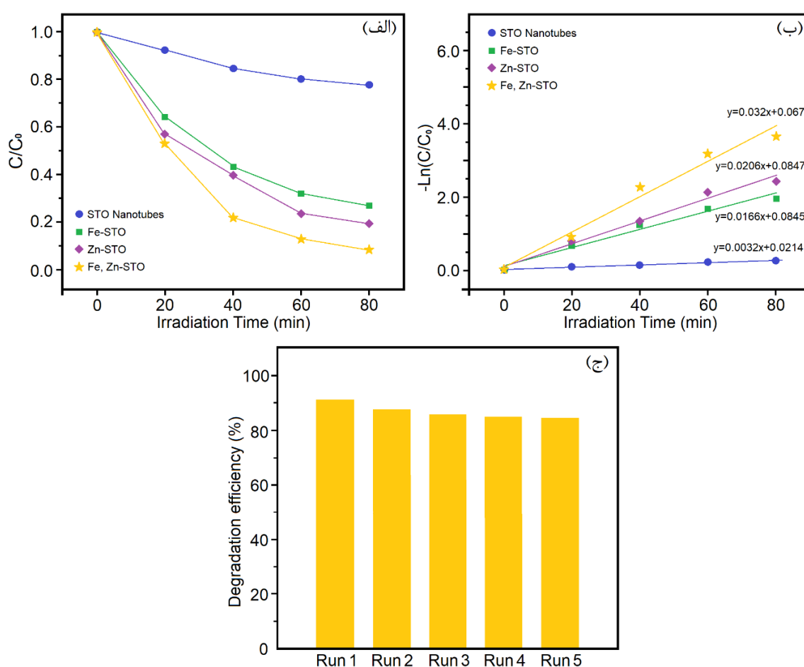
شکل ۳: (الف) تخریب فوتوکاتالیستی نمونه‌های STO، Fe-STO، Zn-STO و Fe برای تخریب رنگ پایه آبی ۴۱ تحت نور مرئی، (ب) منحنی‌های -\ln(C/C_0) بر حسب زمان تابش نور مرئی، (ج) راندمان تخریب فوتوکاتالیستی رنگ پایه آبی ۴۱ در ۵ سیکل متوالی برای نمونه Fe، Zn-STO
