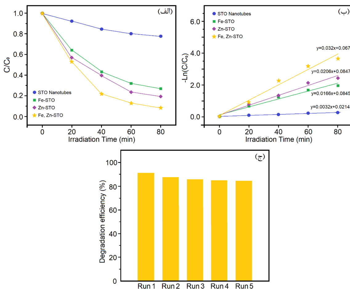
شکل ۳: (الف) تخریب فوتوکاتالیستی نمونه‌های STO، Fe-STO، Zn-STO و Fe، Zn-STO برای تخریب رنگ پایه آبی ۴۱ تحت نور مرئی، (ب) منحنی‌های -\ln(C/C_0) بر حسب زمان تابش نور مرئی، (ج) راندمان تخریب فوتوکاتالیستی رنگ پایه آبی ۴۱ در ۵ سیکل متوالی برای نمونه Fe، Zn-STO
