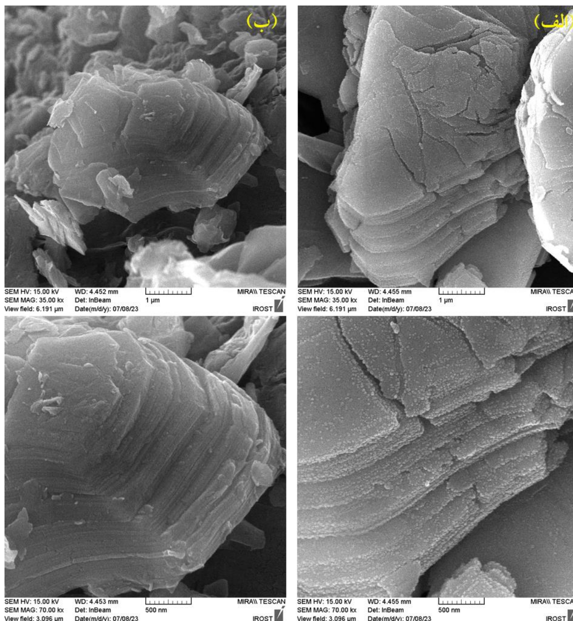
شکل ۳: تصاویر SEM از (الف) پودر مکسین Ti_3C_2Tx فراوری شده به روش حکاکی شیمیایی HF مستقیم و (ب) پودر مکسین Ti_3C_2Tx فراوری شده به روش حکاکی HF درجا (خطوط مقیاس معرف ۵۰۰ نانومتر و ۱ میکرومتر می‌باشند)
