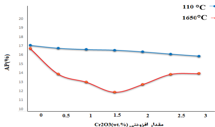
شکل ۴: نتایج مربوط به آزمون میزان تخلخل ظاهری نمونه‌ها در دماهای ۱۱۰ و ۱۶۵۰ °C
