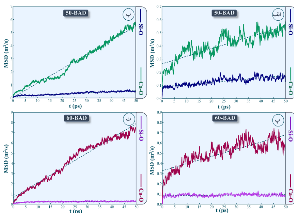
شکل ۵: میانگین مربع جابه‌جایی اتم‌های \text{Si} و \text{Ca} برای ترکیب شیشه‌های زیست‌فعال 50\text{SiO}_2\text{-}50\text{CaO} در دمای الف) 1500\text{ K} و ب) 2000\text{ K} ، برای ترکیب شیشه‌های زیست‌فعال 60\text{SiO}_2\text{-}40\text{CaO} در دمای پ) 1500\text{ K} و ت) 2000\text{ K}
