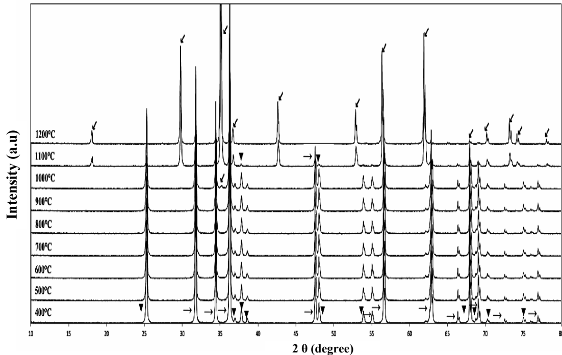
شکل ۵- الگوی پراش اشعه X مربوط به نمونه‌های سنتز شده در مایکروویو در دماهای مختلف؛ ▼: \text{TiO}_2 ، →: \text{ZnO} ، ▲: \text{Zn}_2\text{TiO}_4
