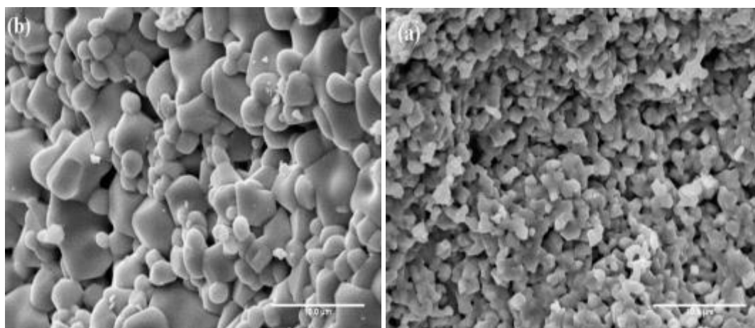
شکل ۷- تصویر SEM ترکیب \text{Zn}_2\text{TiO}_4 سنتز شده در دمای 1200^{\circ}\text{C} (a) میکروویو (b) کوره الکتريکی
