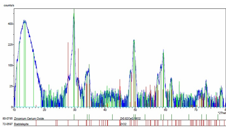
شکل ۳- نمونه ۲: زیرکونیای پایدار شده با سربیم در دمای ۱۵۵۰ درجه سانتیگراد [۴].
