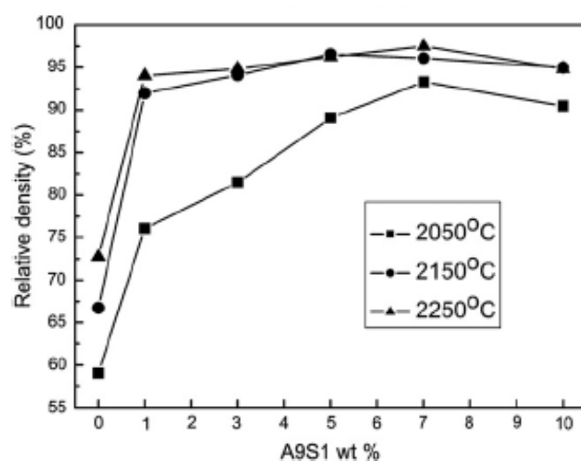
شکل ۲- تغییرات دانشیته نمونه‌های سینتر شده در دماهای سینتر ۲۰۵۰، ۲۱۵۰ و ۲۲۵۰ درجه سانتی گراد [۱۴].
