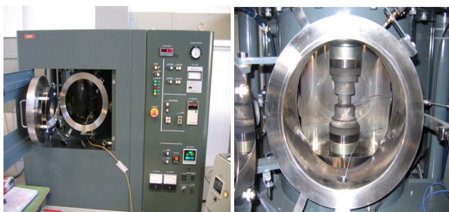
شکل ۲- محفظه خلأ و محور اعمال فشار [9]
