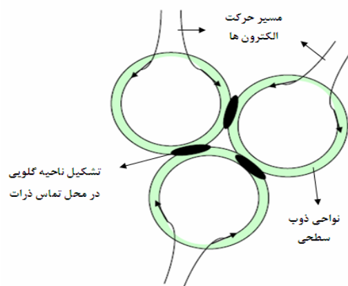
شکل ۵- حرارت موضعی ایجاد شده در محل تماس ذرات پودر بر اثر تخلیه الکتریکی (ذوب سطحی) و تشکیل ناحیه گلوئی [11]
