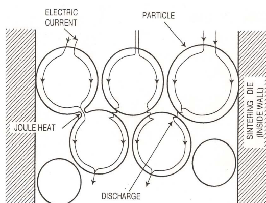
شکل ۴- تصویر شماتیک عبور پالس‌های جریان از میان ذرات پودر و تولید حرارت (تشکیل ناحیه گلوئی) [5,7]
