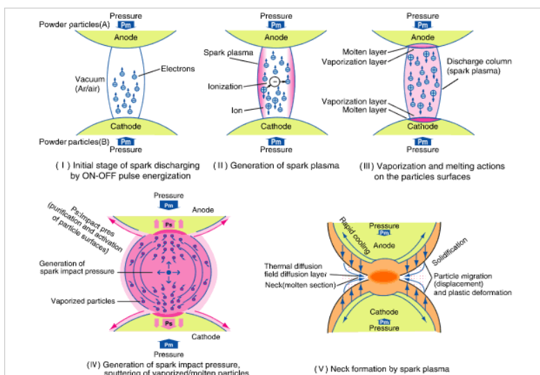
شکل ۶- مراحل تشکیل ناحیه گلوئی [5]
