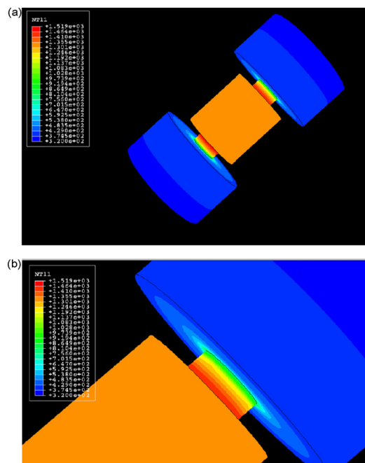
شکل ۱۴- شبیه‌سازی توزیع دما در سطح قالب و پانچ‌ها پس از گذشت ۴۵۰ ثانیه از فرآیند SPS: (a) شمای کلی مجموعه قالب/پانچ/صفحه گرافیتی و (b) قسمت بالایی پانچ و محل اتصال پانچ/صفحه گرافیتی [12]
