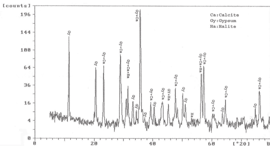
شکل ۱۳- پراش پرتو ایکس سنگ‌های فرسایش یافته دارای فازهای کلسیت، سولفات کلسیم (ژیپس) و هالیت
