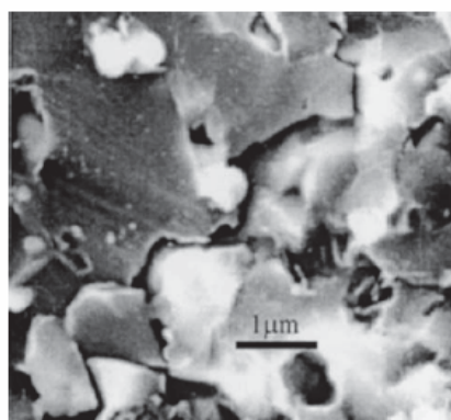
شکل ۵- شکست بین دانه‌ای در کامپوزیت ایجاد شده، افزایش استحکام را در پی دارد [۲۶].
