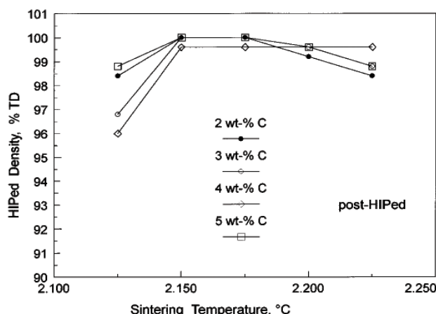
شکل ۱- نمودار تغییرات دانسیته نسبی قطعات حاوی کمک زینتر کربن، زینتر شده به روش پرس ایزو استاتیک گرم در فشار ۲۰۰ MPa بر حسب دما و درصد کربن [۱۸].
