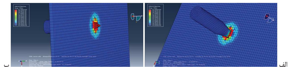
شکل ۱۱- لحظه برخورد نفوذگر به هدف در زمان 0.006 ثانیه (الف) از نمای جلوی هدف، (ب) از نمای پشت هدف
