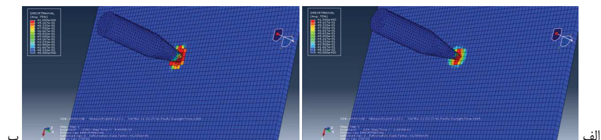
شکل ۱۰- لحظه برخورد نفوذگر به هدف (الف) در زمان 0.002 ثانیه، (ب) در زمان 0.004 ثانیه
