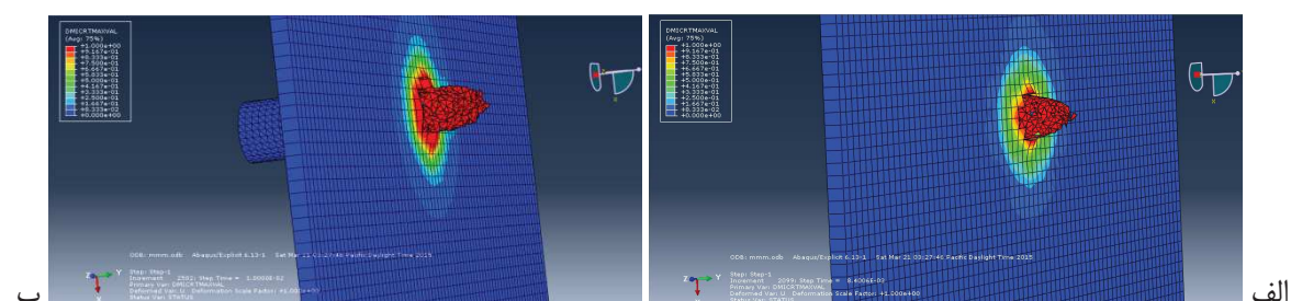
شکل ۱۲- لحظه برخورد نفوذگر به هدف از نمای پشت هدف (الف) در زمان 0.008 ثانیه، (ب) در زمان 0.01 ثانیه
