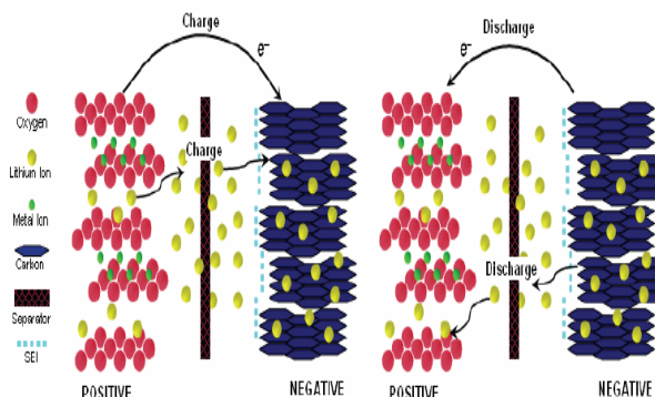
شکل ۱- مکانیزم واکنش‌های شارژ و تخلیه باتری‌های لیتیم-یون [۳]
