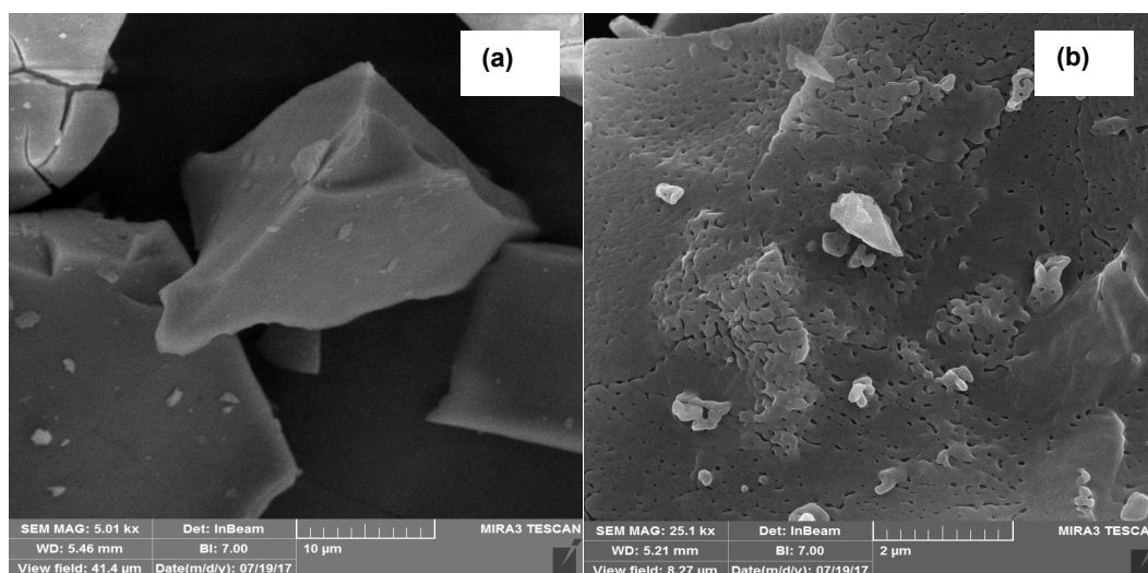
شکل ۲- تصاویر FESEM نانوذرات \text{Al}_2\text{O}_3 (a) نمونه خالص، (b) نمونه‌های آلائیده شده با آهن ۳٪
