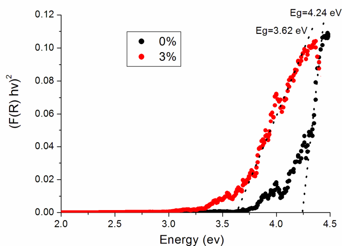
شکل ۴- منحنی تائوک نمونه‌های خالص و ناخالص برای محاسبه گاف نواری
