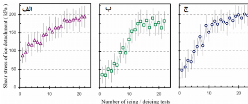
شکل ۱۴- استحکام چسبندگی یخ به عنوان تابعی از چرخه یخ زدگی/یخ زدایی بر روی سه سطح فوق آبگریز: پوشش دهی دورانی ZrO_2 ترکیب شده با فلوئوروپلیمر (الف)، FAS-17 (ب) و آلومینیم اچ شده پوشش داده شده با اسید استاریک (ج) [۲۱].
