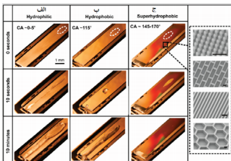
شکل ۸- انباشتگی یخ بر روی سطح صاف آلومینیم آبدوست (الف)، سطح صاف سیلیسیم فلئوئوردار آبگریز (ب) و سطح میکرو ساختار فوق آبگریز سیلیسیم فلئوئوردار (ج). مقادیر زاویه تماس با توجه به زاویه تماس پیشروی قطرات آب بر روی هر سطح اندازه گیری شده است. [۲۰].
