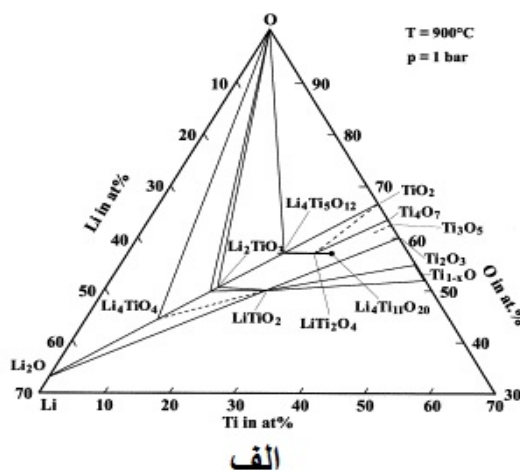
شکل ۲- (الف) دیاگرام سه‌تایی Li-Ti-O (ب) نمودار فازي سیستم \text{Li}_2\text{O}-\text{TiO}_2 [۳]
