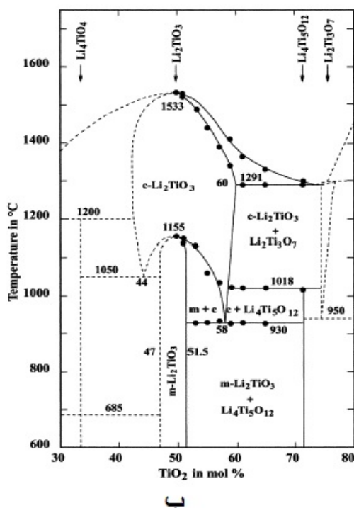
شکل ۲- (الف) دیاگرام سه‌تایی Li-Ti-O (ب) نمودار فازي سیستم \text{Li}_2\text{O}-\text{TiO}_2 [۳]
