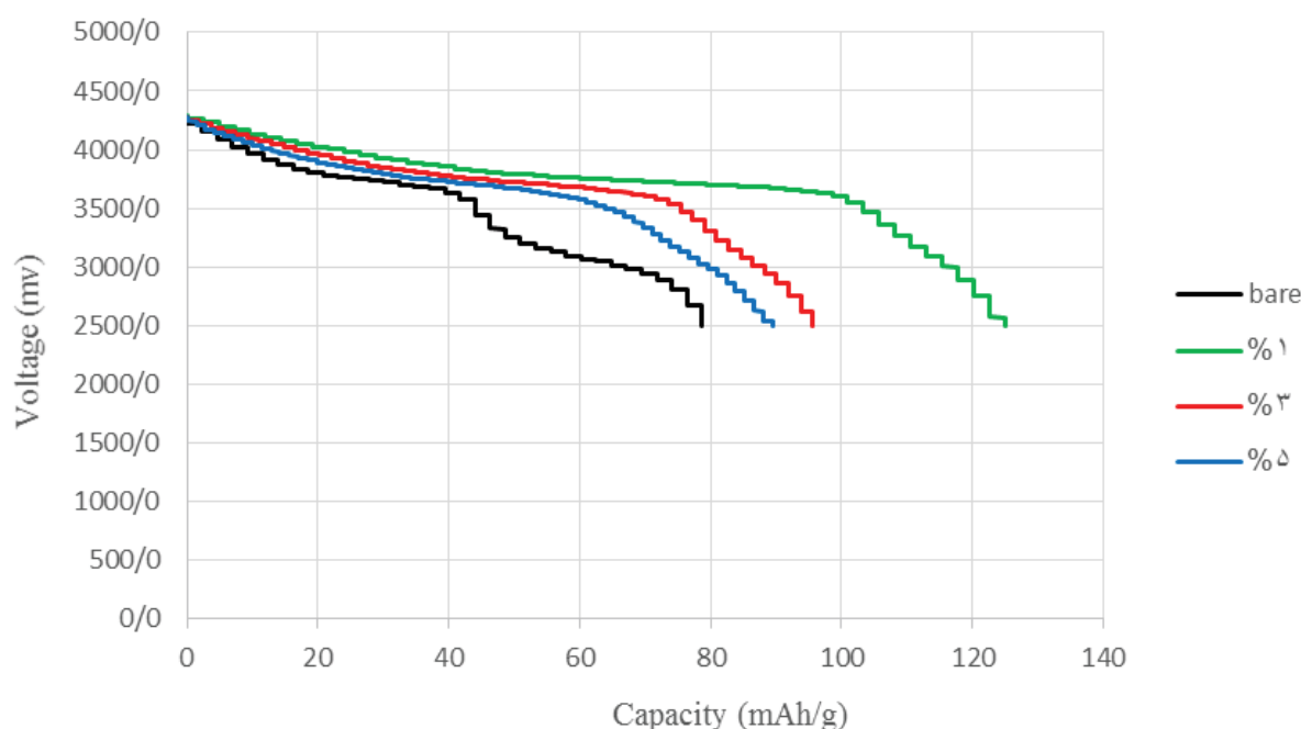
شکل ۳- نمودار ولتاژ بر حسب ظرفیت در فرآیند تخلیه نمونه ماده کاتدی LiNi_{0.5}Co_{0.2}Mn_{0.3}O_2 بدون پوشش و پوشش داده شده با ۱٪ وزنی، ۳٪ وزنی و ۵٪ وزنی از ماده پوشش لیتیم زیرکونات با سرعت تخلیه ۰.۰۵ C
