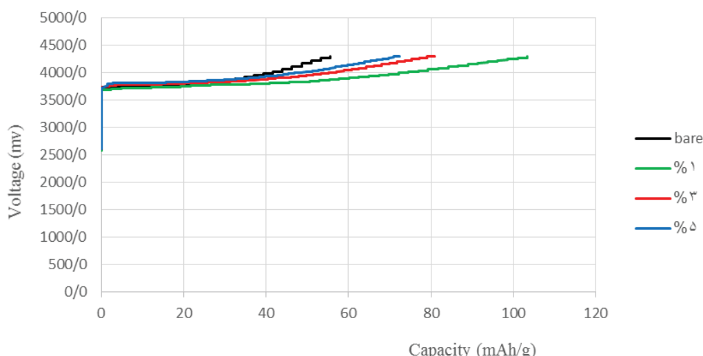
شکل ۴- نمودار ولتاژ بر حسب ظرفیت در فرآیند تغذیه نمونه ماده کاتدی \text{LiNi}_{0.5}\text{Co}_{0.2}\text{Mn}_{0.3}\text{O}_2 بدون پوشش و پوشش داده شده با ۱٪، ۳٪، ۵٪ وزنی از ماده پوشش لیتیم زیرکونات با سرعت تغذیه ۰.۱، ۰.۳، ۰.۵ و ۱.۰ V/s.
