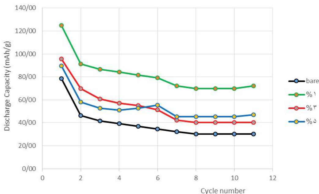
شکل ۸ - نمودار ظرفیت تخلیه بر حسب تعداد سیکل کاری باتری برای نمونه ماده کاتدی \text{LiNi}_{0.5}\text{Co}_{0.2}\text{Mn}_{0.3}\text{O}_2 بدون پوشش و پوشش داده شده با ۱٪ وزنی، ۳٪ وزنی و ۵٪ وزنی از ماده پوشش.
