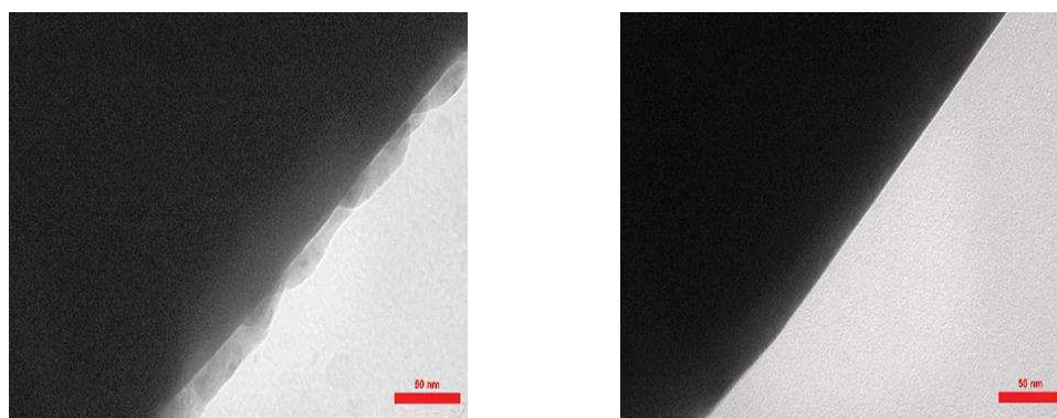
شکل ۱- تصاویر میکروسکوپ الکترونی عبوری در مقیاس ۵۰ نانومتر (الف) نمونه ماده کاتدی بدون پوشش و (ب) نمونه ماده کاتدی پوشش داده شده با ۱٪ وزنی ماده پوشش.
