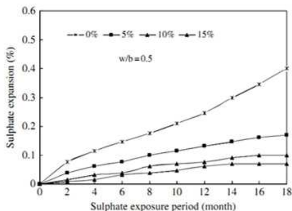
شکل ۱۳- اثر متاکائولن روی تغییرات انبساط ناشی از حمله سولفات‌ها (نسب آب/چسب ۰/۵) [۲۳]
