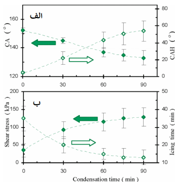
شکل ۱۵- (الف) مقادیر زاویه تماس (CA) و پسماند زاویه تماس (CHA) بر روی سطح فوق آبریز پوشش داده شده FAS-17 به عنوان تابعی از زمان میعان آب. (ب) تنش برشی جدا شدن یخ (لوزی توپر) و زمان یخ زدگی (لوزی توخالی) بر روی همان سطح به عنوان تابعی از زمان میعان آب [۲۱].
