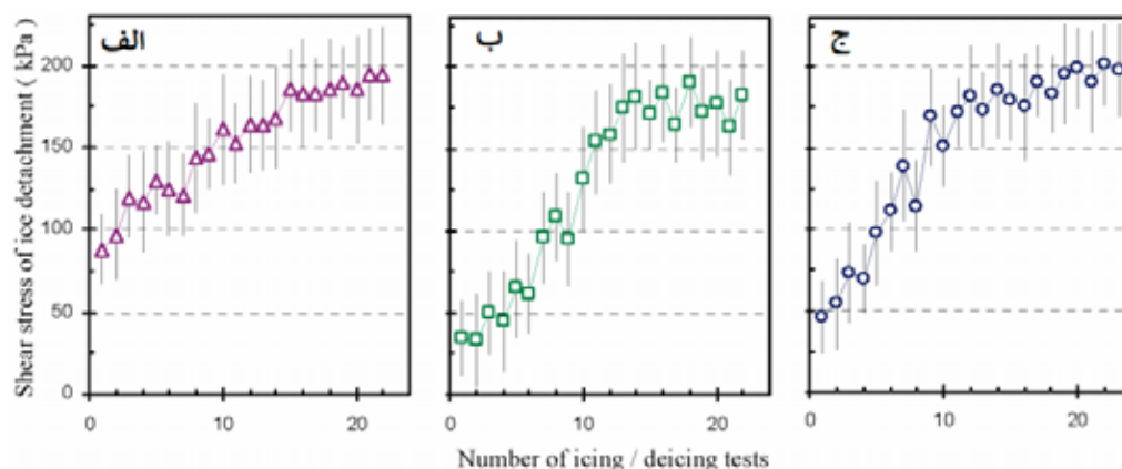
شکل ۱۴- استحکام چسبندگی یخ به عنوان تابعی از چرخه یخ زدگی/یخ زدایی بر روی سه سطح فوق آبریز: پوشش دهی دورانی ZrO_2 ترکیب شده با فلوئوروپلیمر (الف)، FAS-17 (ب) و آلومینیم اچ شده پوشش داده شده با اسید استاریک (ج) [۲۱].
