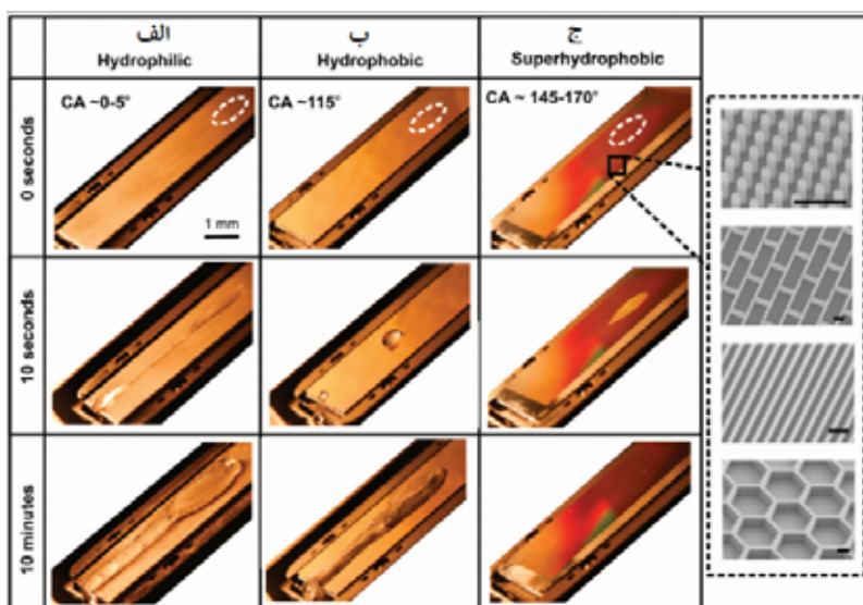
شکل ۸- انباشتگی یخ بر روی سطح صاف آلومینیم آبدوست (الف)، سطح صاف سیلیسیم فلئوئردار آبگریز (ب) و سطح میکرو ساختار فوق آبگریز سیلیسیم فلئوئردار (ج). مقادیر زاویه تماس با توجه به زاویه تماس پیشروی قطرات آب بر روی هر سطح اندازه گیری شده است. [۲۰].
