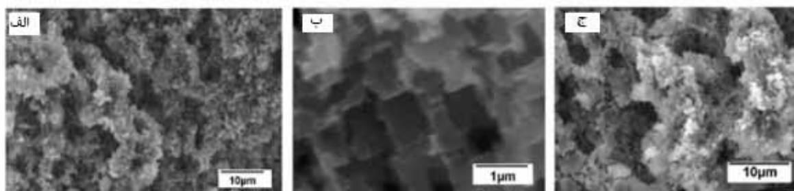
شکل ۷- تصاویر میکروسکوپ الکترونی روبشی سطح آلومینیم فوق آبگریز در بزرگنمایی مختلف [۱۹].
