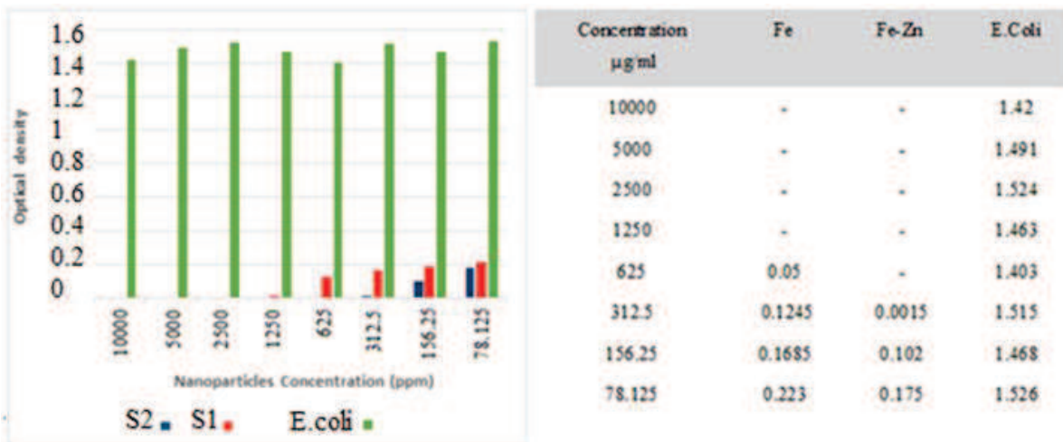
شکل ۶- نمودار و نتایج مربوط به خاصیت ضد باکتری نانوذرات سنتز شده در برابر باکتری E.coli.
