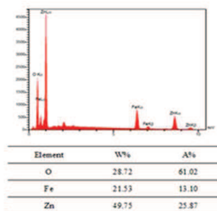
شکل ۴- تصویر FESEM و نمودار توزیع فراوانی اندازه ذرات و تصویر EDS مربوط به نمونه S2.
