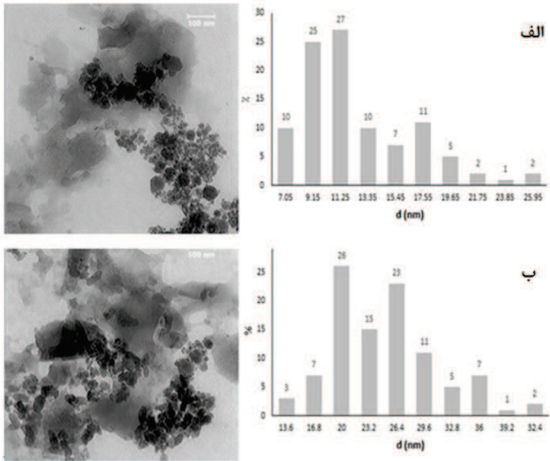
شکل ۵- الف) تصویر TEM و نمودار توزیع اندازه ذرات مربوط به نمونه S1، ب) تصویر TEM و نمودار توزیع اندازه ذرات مربوط به نمونه S2.
