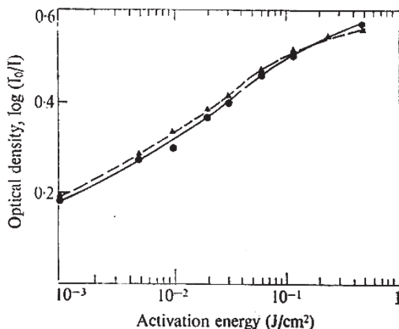
شکل ۶- بررسی خستگی نوری در شیشه های کادمیوم بوروسیلیکات [۱۵]
