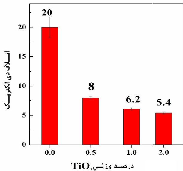
شکل ۵- تغییرات اتلاف دی الکتریک ZnO بر حسب مقدار افزودنی TiO_2 .
